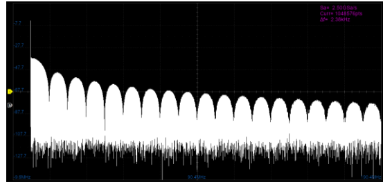
频谱仪模式
