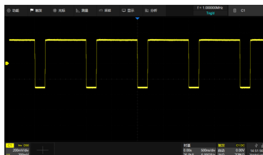
反相开启
