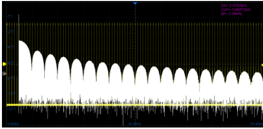
全屏模式
